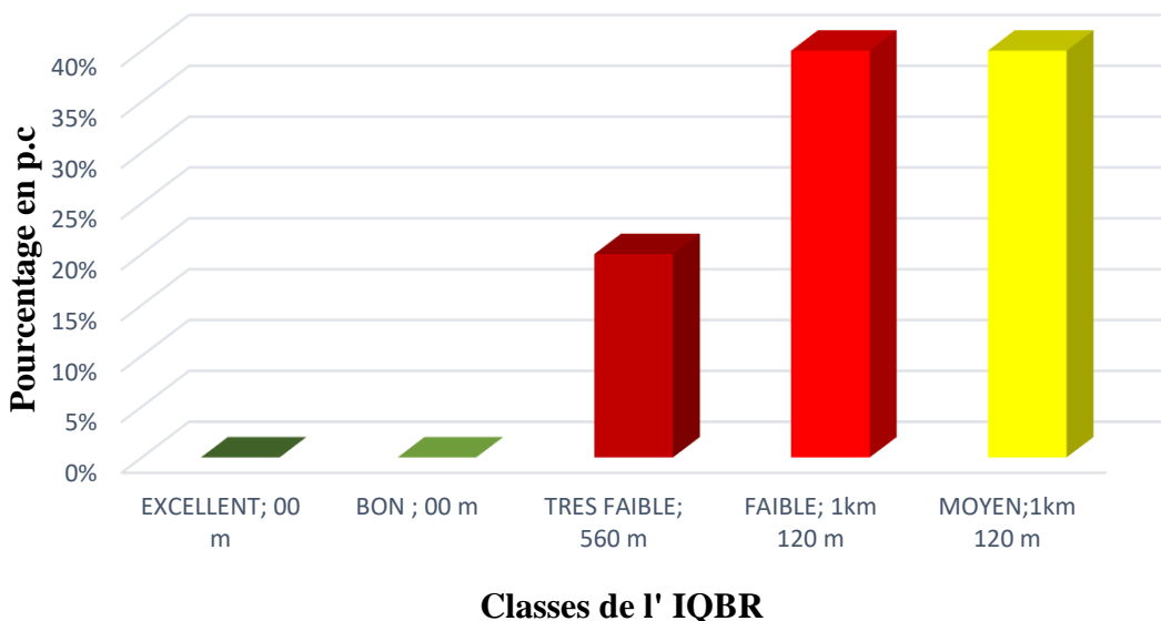
Fig. 5. Proportions des classes de qualité de bande riveraine de la rive gauche
