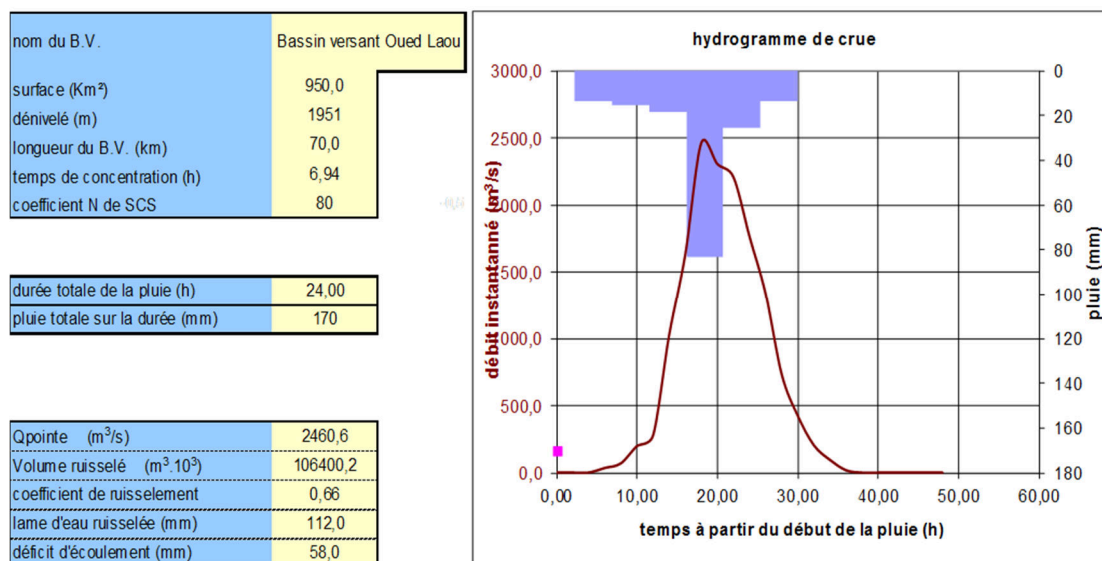
Fig. 5. Hydrogramme de crue du bassin versant de Oued Laou calculé par la méthode SCS
